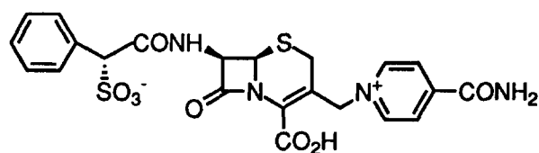
cefsulodin
