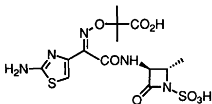
aztreonam
