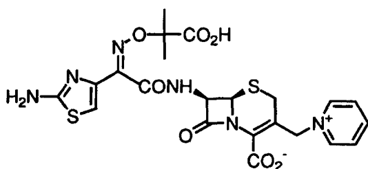
ceftazidime
