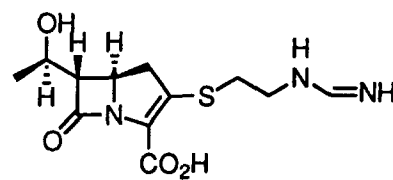
imipenem
